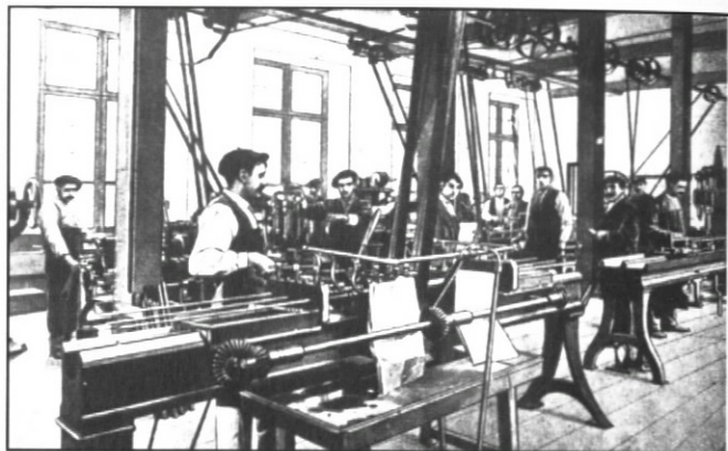
Perforación y barrenado de cañones a principios de siglo en la empresa eibarresa Víctor Sarasqueta, Cortaberría y Cía.
