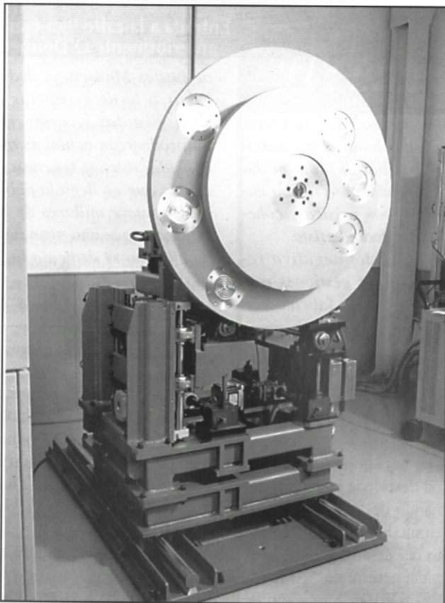
Difractómetro de rayos X, desarrollado por Tekniker para el sincrotrón de Grenoble.
