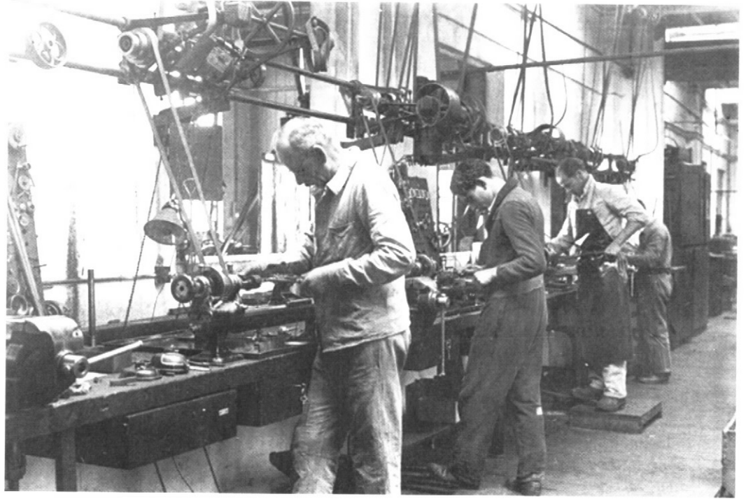
Operaciones de limado en la fabricación de quemadores de petróleo.
