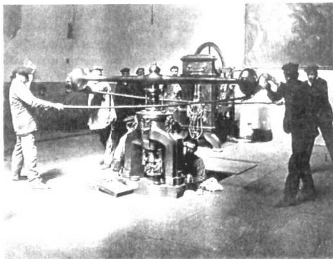
Prensa de balancín, en la Casa de Moneda de Madrid.
