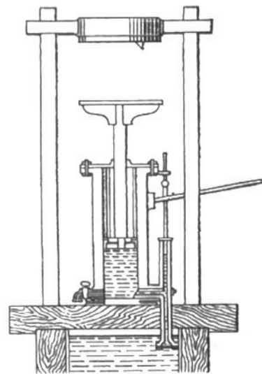
Año 1812. Prensa hidráulica de los Hnos. Perier.
