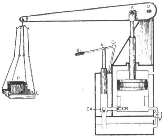
Año 1770. Prensa hidráulica de Joseph Bramah.
