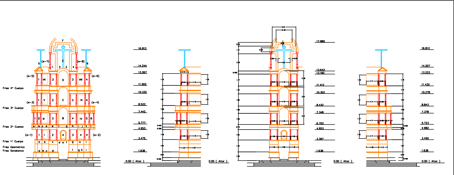
ALZADO
