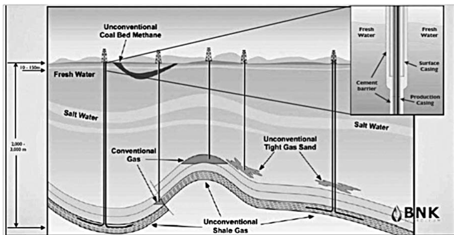
** Esquema de los diferentes tipos de yacimientos de Hidrocarburos. Obtenido del Informe del Consejo superior de Colegios de Ingenieros de Minas “Gas no convencional en España. Una oportunidad de futuro”. Se puede acceder a este informe por internet.
