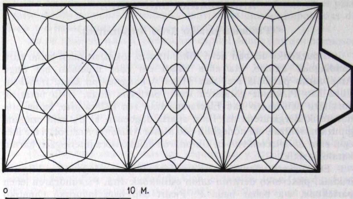
Angiozarko San Migel elizaren sabai estruktura. (Gipuzkoa).
